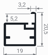
MZ 07 Профиль фасадный
