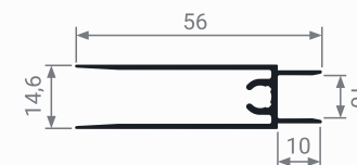
MS 220C Профиль горизонтальный нижний
