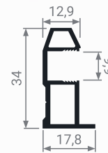
MS 161 Профиль вертикальный
