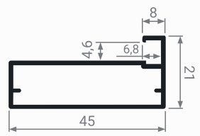
MZ 13 Профиль фасадный
