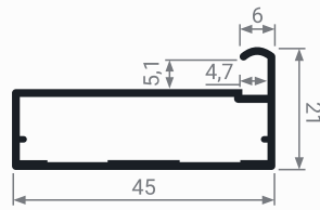
MZ 09 Профиль фасадный
