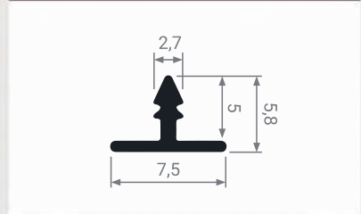
T-08 Профиль разделительный декоративный врезной
