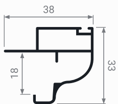
MS 50 Профиль вертикальный
