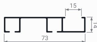
MS 52 Направляющая верхняя
