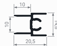
MS 210C Профиль горизонтальный верхний
