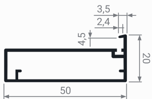
MZ 17 Профиль фасадный
