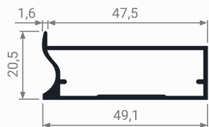
MZ 19 Профиль фасадный
