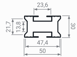
РА 01 Профиль опорный алюминиевый
