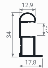
MS 162 Профиль вертикальный
