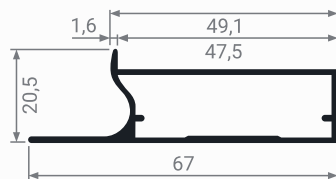
MZ 20 Профиль фасадный
