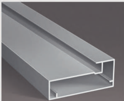
MZ 04 Профиль фасадный
