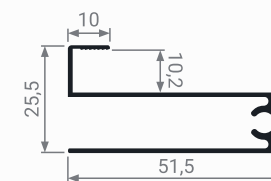
MS 225 Профиль горизонтальный нижний
