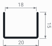
MS 51 Профиль горизонтальный
