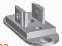
PP 02 Крепление пол-потолок с площадкой под саморез
