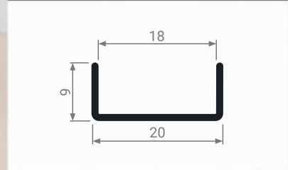
C18-02 Профиль фасадный
